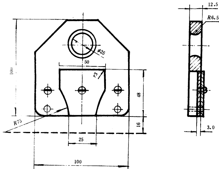
图 1 III 型试样夹具
